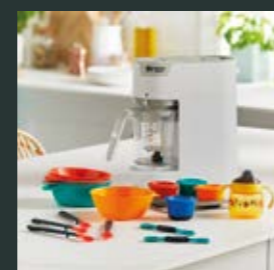
PRIMEROS SÓLIDOS
